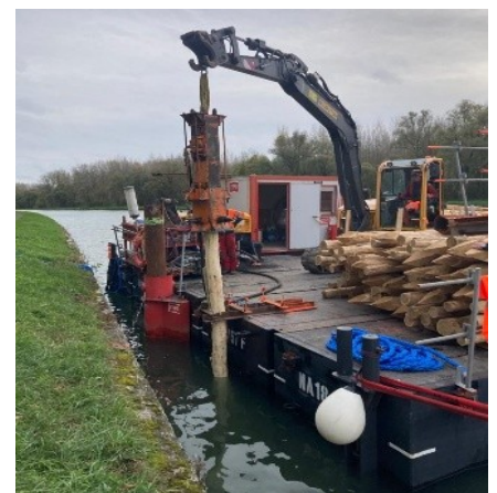
Uferbefestigung
