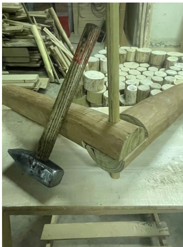
Îmbinare cu dibluri
