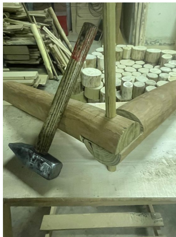
Dübelverbindung
