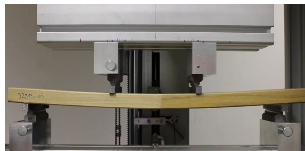
Teste de rezistență efectuate în laborator (UCL – Belgia)
